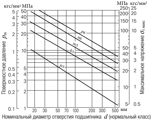
Рис.15.5. Поверхностное давление p_m , а также максимальное напряжение \sigma_{T \text{ макс}} для среднего натяга
