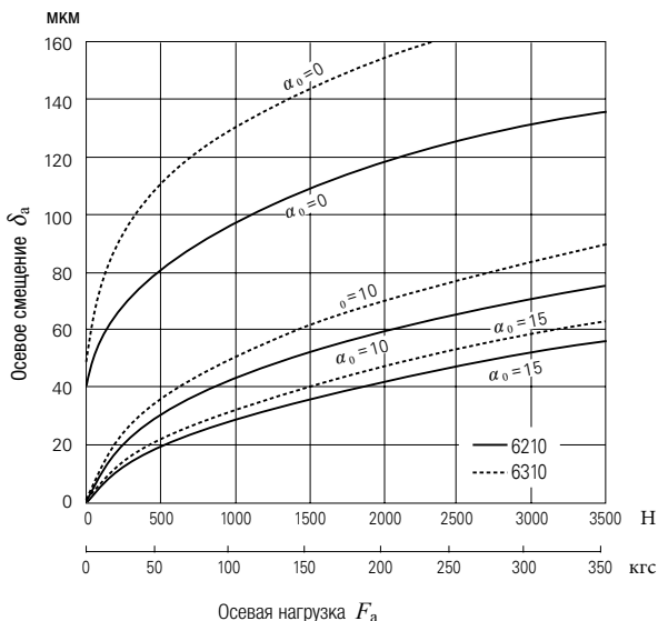
Рис. 15.2. Осевая нагрузка и осевое смещение радиальных шарикоподшипников
