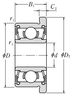
С контактнм уплотнением DD
