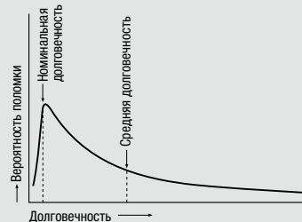
Рисунок 5.2. Вероятность поломки и долговечность подшипника
